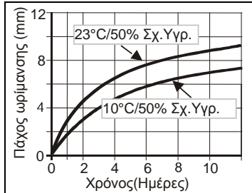
Διάγραμμα 1: Ταχύτητα ωρίμανσης Sikaflex®-298
